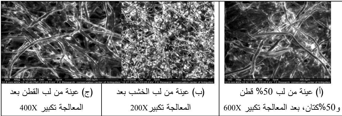
اللوحة رقم (7) تأثير المعالجة الكيميائية باستخدام الكحول الإيثيلي في العينات الورقية المصابة بالفطريات تحت المجهر الإلكتروني الماسح
