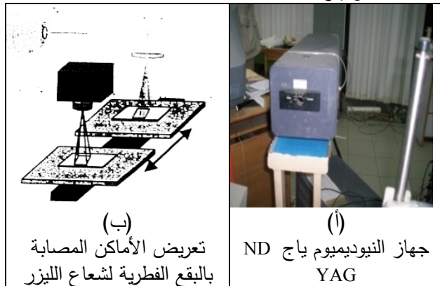
اللوحة رقم (8). جهاز الليزر المستخدم في تنظيف البقع الفطرية
