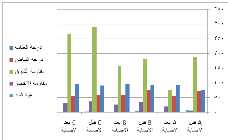
شكل (1). يوضح قياس الخواص الضوئية والميكانيكية لأنواع المختلفة من الأوراق قبل وبعد الإصابة بالفطريات
