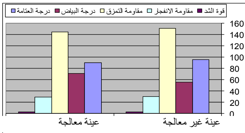
الشكل رقم (3): قياس الخواص الميكانيكية والضوئية للأوراق المعالجة بأشعة الليزر
