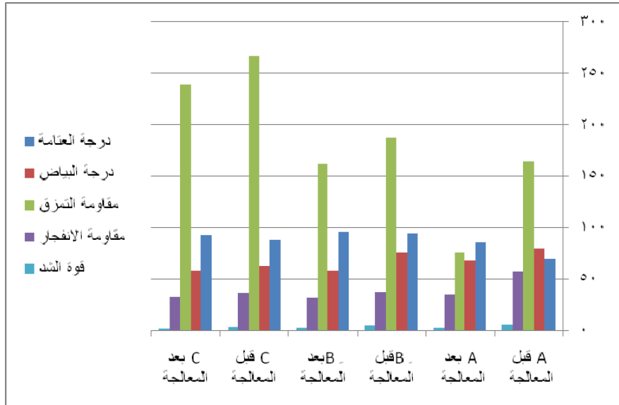
الشكل رقم (2). تأثير التنظيف بالكحول الإيثيلي 5% في الخواص الميكانيكية والضوئية للورق
